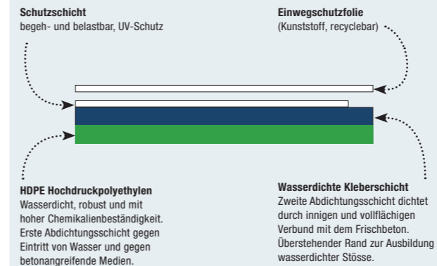
Wandflächenabdichtung zum Beispiel bei Schlitzwänden oder Unterfangungen.
